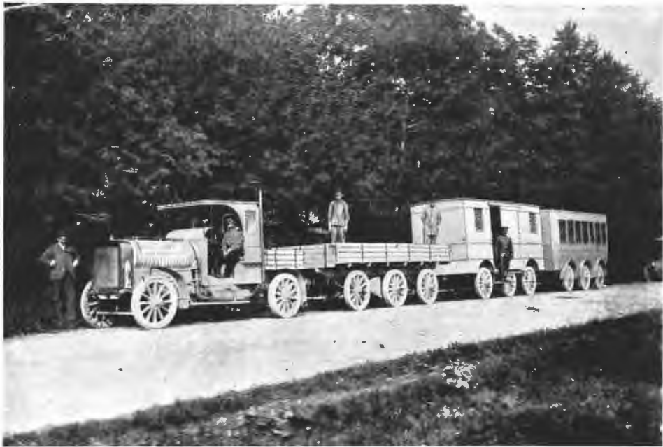
Багажный моторъ для перевозки тяжестей. Моторъ этотъ съ успѣхомъ испытывался на послѣднихъ маневрахъ въ Красномъ Селѣ въ качествѣ обоза военнаго времени.
