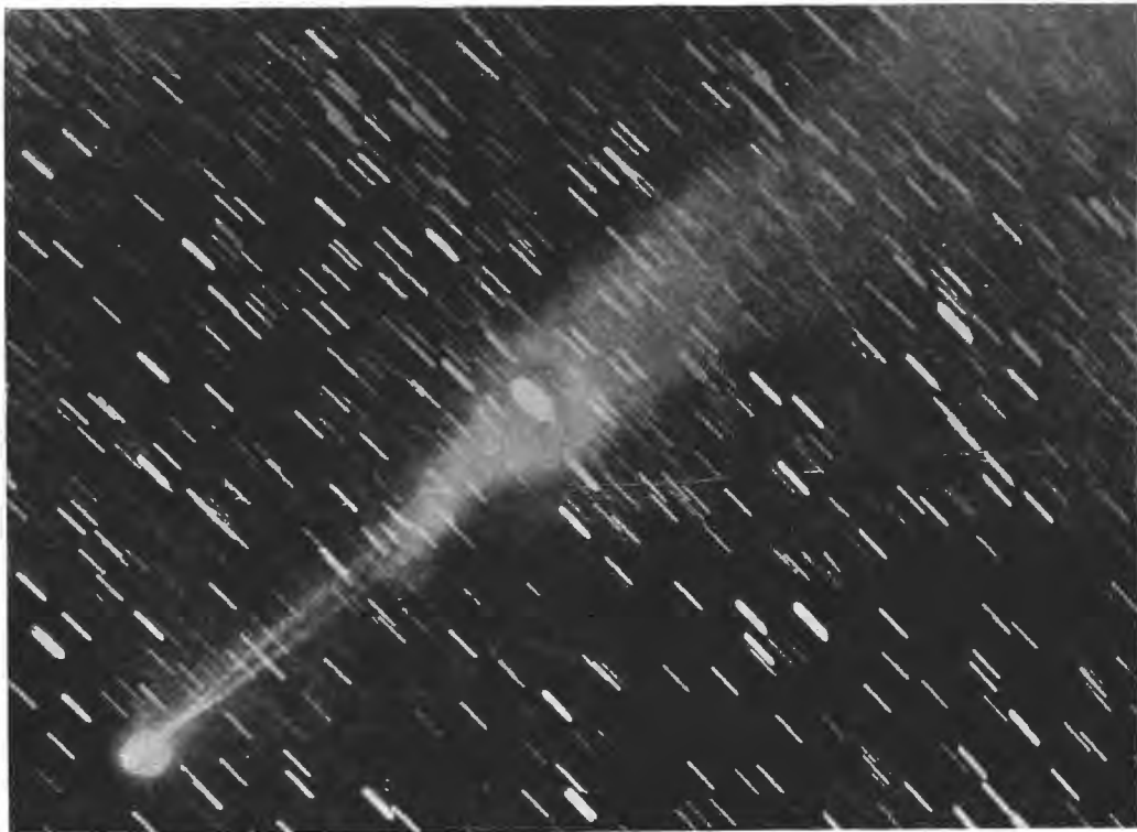
Комета Морхауза-Борелли. Рѣдная фотографія кометы. По снимку кометы Морхауза-Борелли, исполненному въ обсерваторіи Жювизи.
