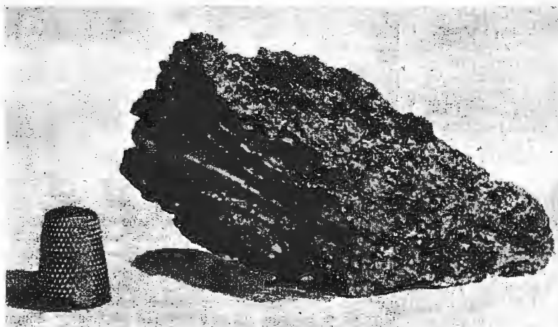
«Лондонскій дымъ». Глыба угольной копоти на кровлѣ собора св. Павла въ Лондонѣ.
