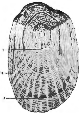
Рис. 1. Чешуйка камбалы (по Майеру). Цифры 1, 2, 3 указываютъ границы годового прироста. Увеличено въ 25 разъ.
