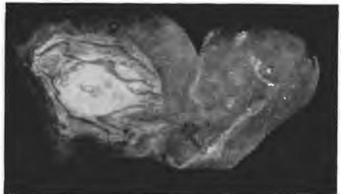
Двойная градина, сфотографированная слегка уже обтаявшей.
