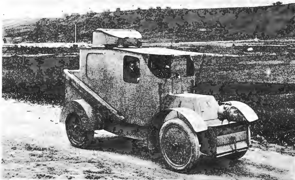
Блиндированный автомобиль системы кн. М. А. Накашидзе. Въ пути.
