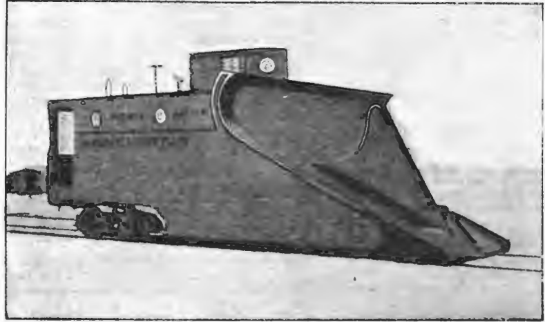
Борьба со снежными заносами. Снегоочиститель «The Russell».
