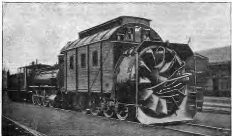
«Борьба со снежными заносами». Механический ротативный снегоочиститель.
