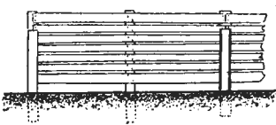
Деревянные загородки для защиты пути от снежных заносов.
