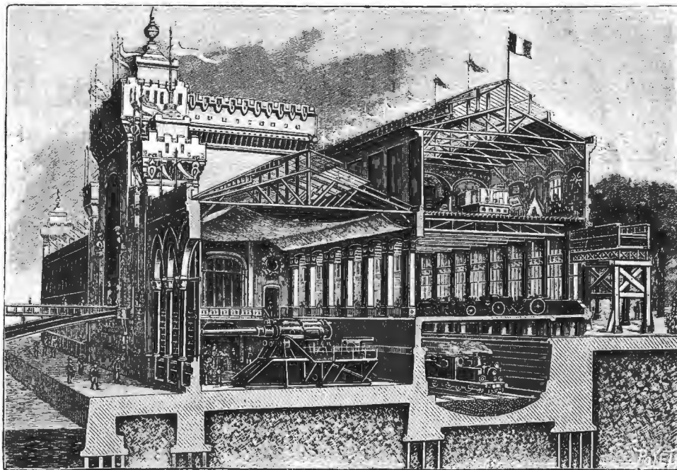
Парижская всемірная выставка 1900 г. Дворецъ Арміи и Флота (въ разрѣзѣ).
