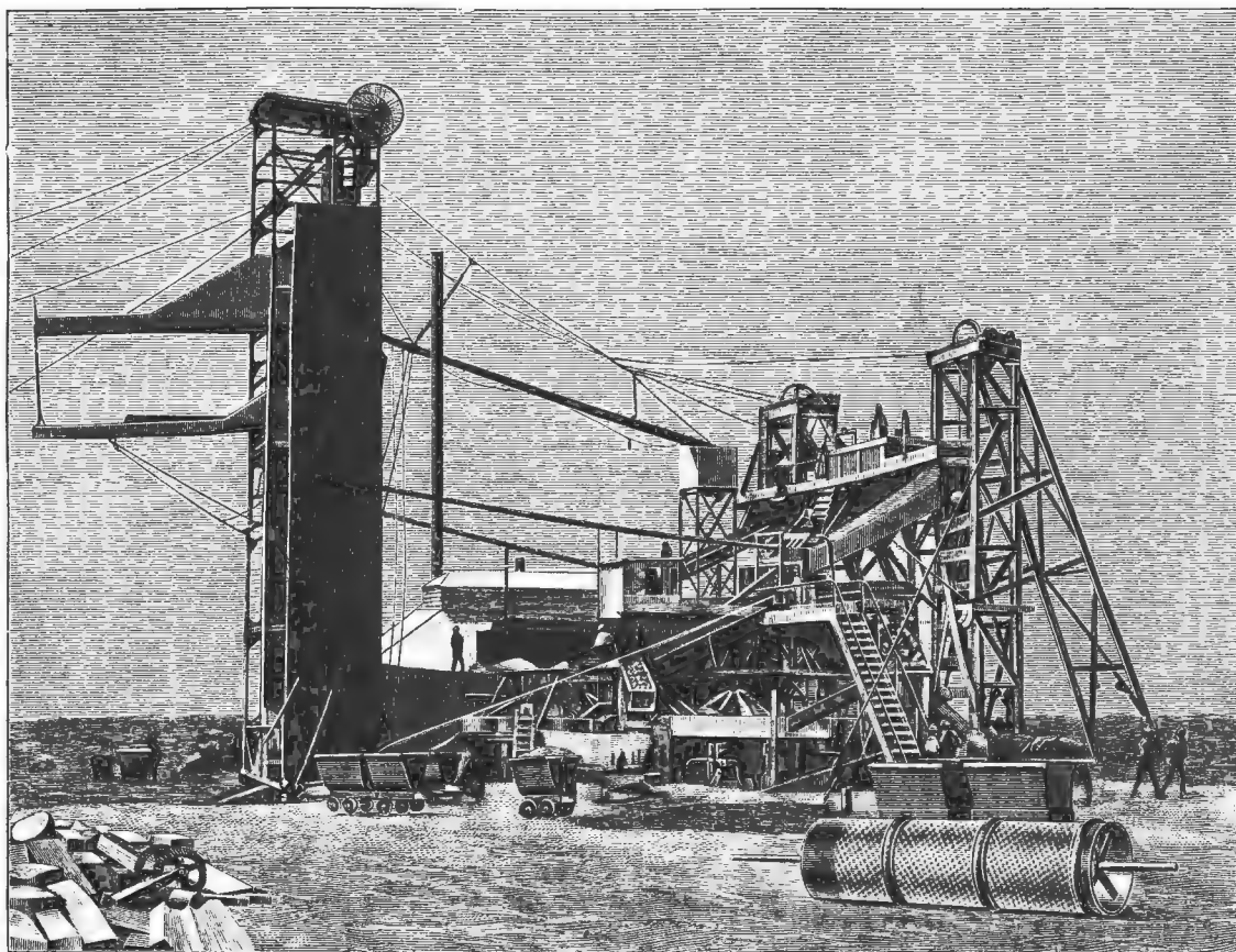
Алмазные копи в Кимберлеѣ. Машина для промывки алмазо-содержащей массы. По фот. грав. Бонгъ.
