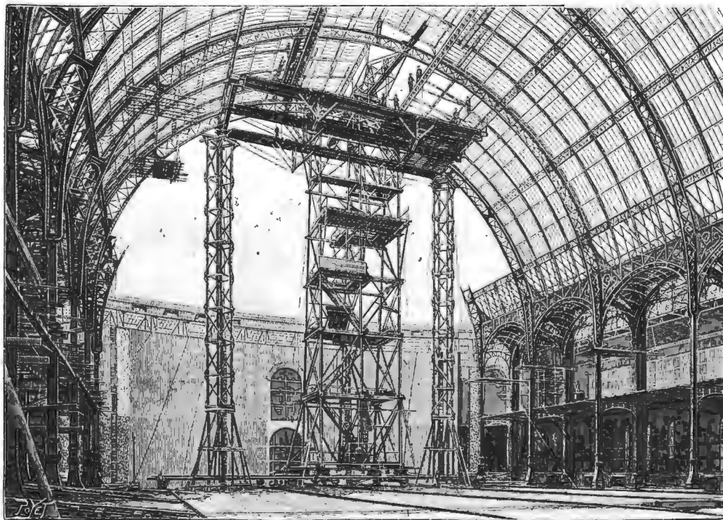
Парижская всемірная выставка 1900 г. Работы по возведенію Большаго дворца искусствъ. Средніе лѣса.
