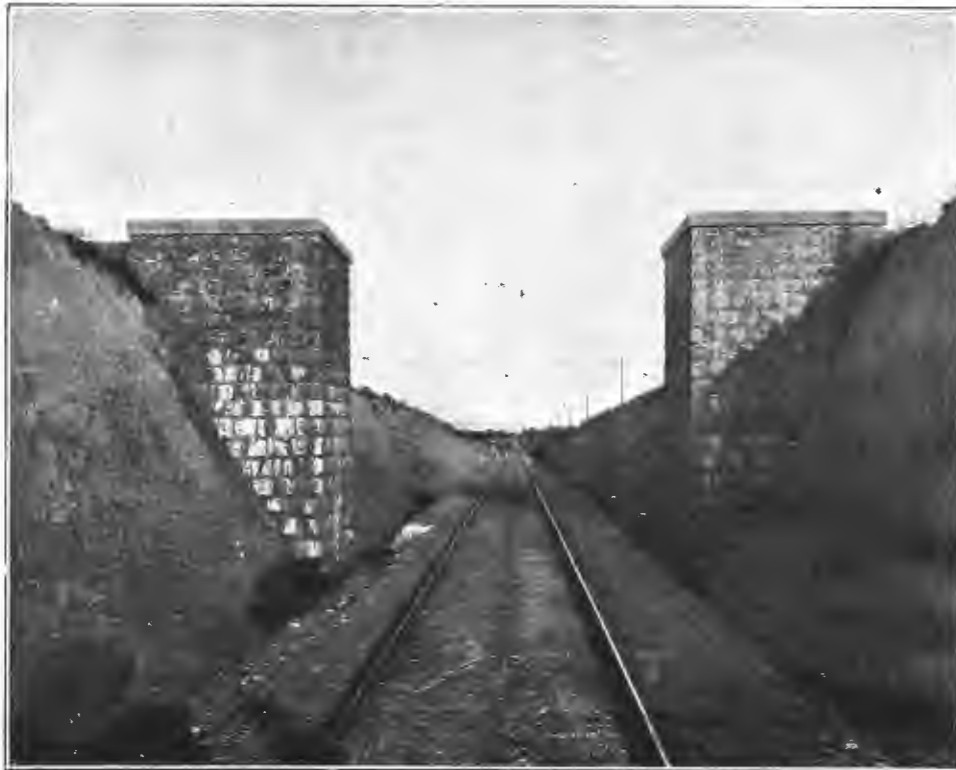
Сифонъ для пропуска оросительной канавы (арыка), на 230-ой верстѣ.
