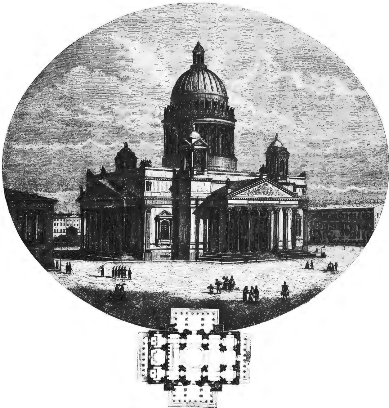
Фасадъ и планъ Исаакиевскаго собора.
