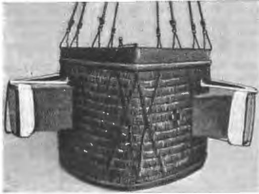
Приспособленіе гондолы аэростата для плаванія. Воздушныя камеры, поддерживающія корзину аэростата на водѣ, какъ плавательныя пузыри.
