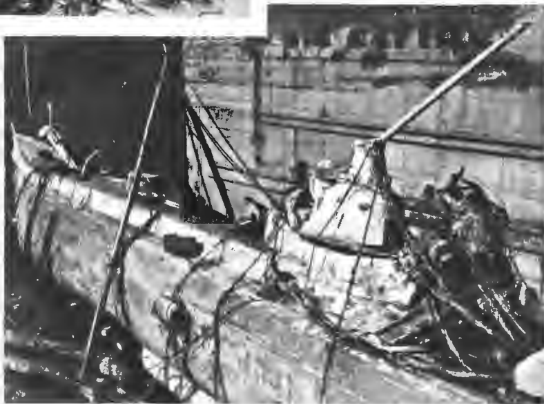
Носовая часть лодки „Камбала“ съ боевой рубкой, погнутымъ перископомъ и открытымъ входнымъ люкомъ (а), черезъ который были извлечены трупы погибшихъ.
