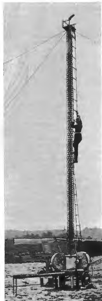
Стальная раздвижная колонна Сиверса въ развернутомъ видѣ, съ лѣстницею.
