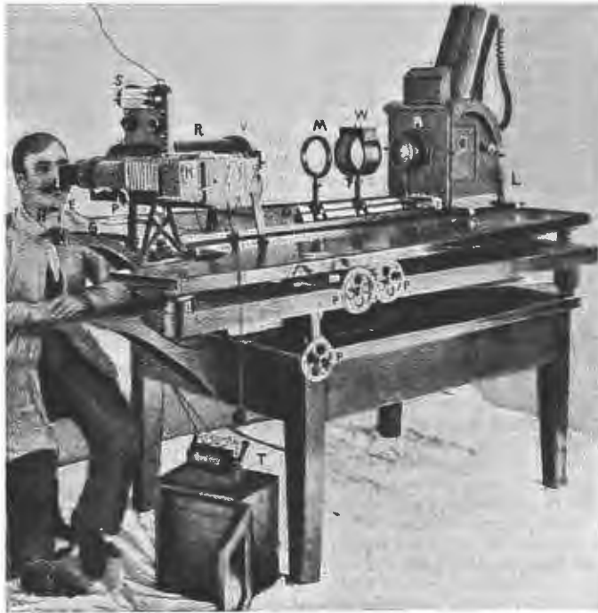
Аппаратъ для фотографированія глазного дна.
