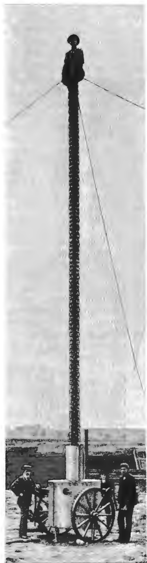
Стальная раздвижная колонна Сиверса въ развернутомъ видѣ, съ вышкой и часовымъ на вершинѣ.
