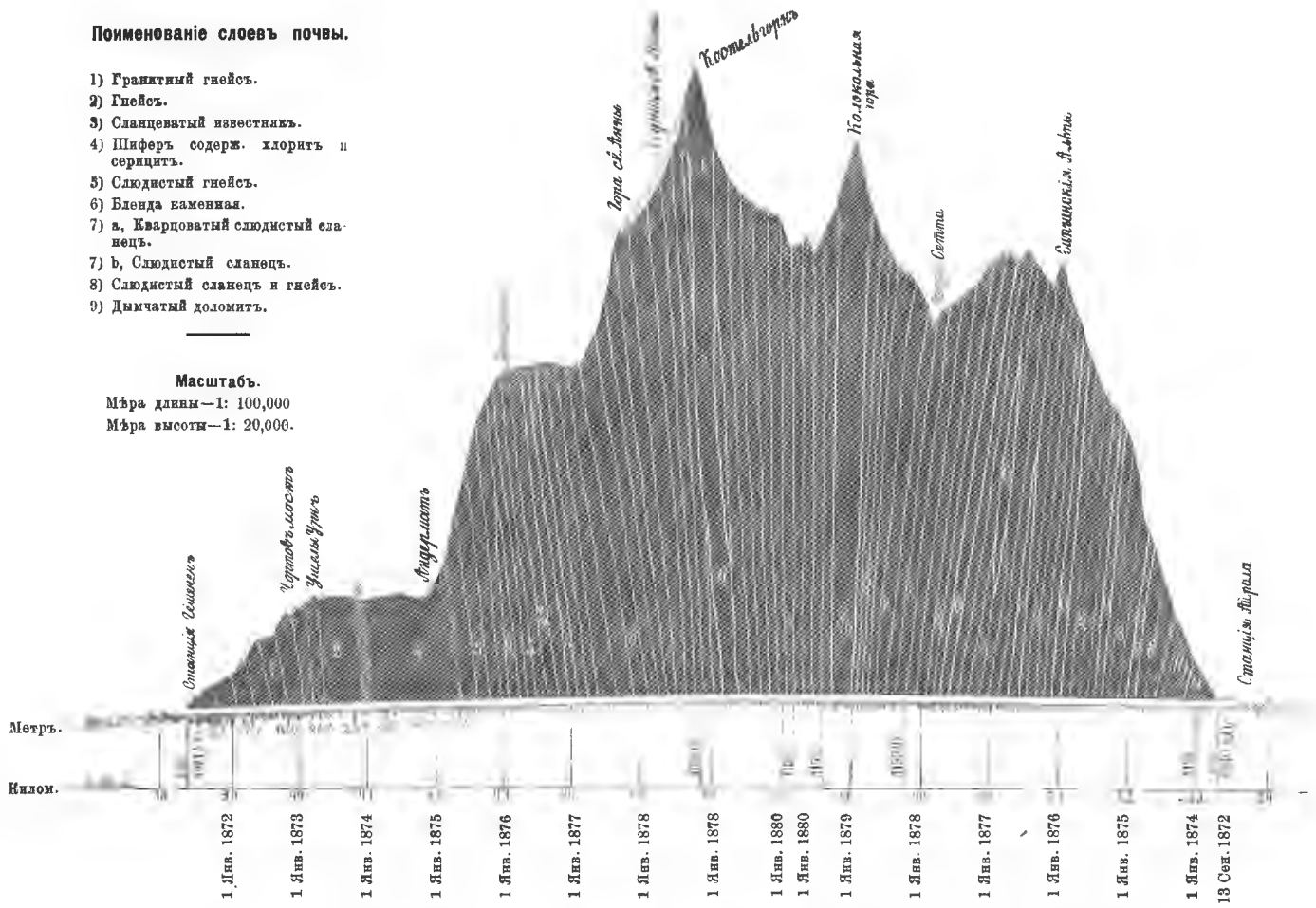
Разрѣзъ горы С. Готарда и туннеля, для показанія слоевъ почвы Рис. Фарскій, грав. Э. Шмидтъ.
