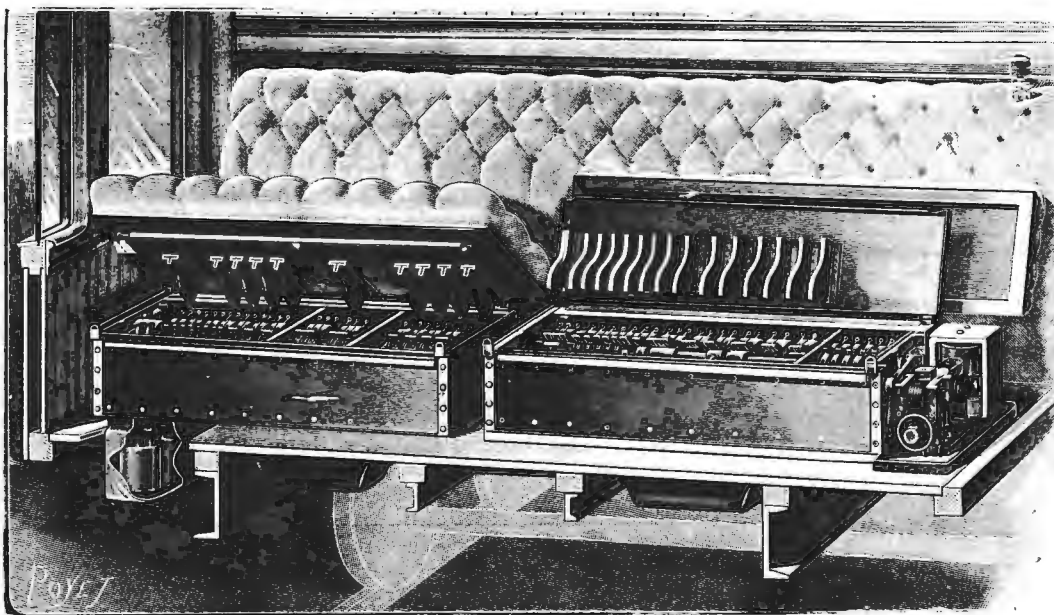
Новая система электрическихъ поездовъ. Рис. 3. Инверсоръ и регуляторъ, устроенные подъ сидѣньемъ вагона.
