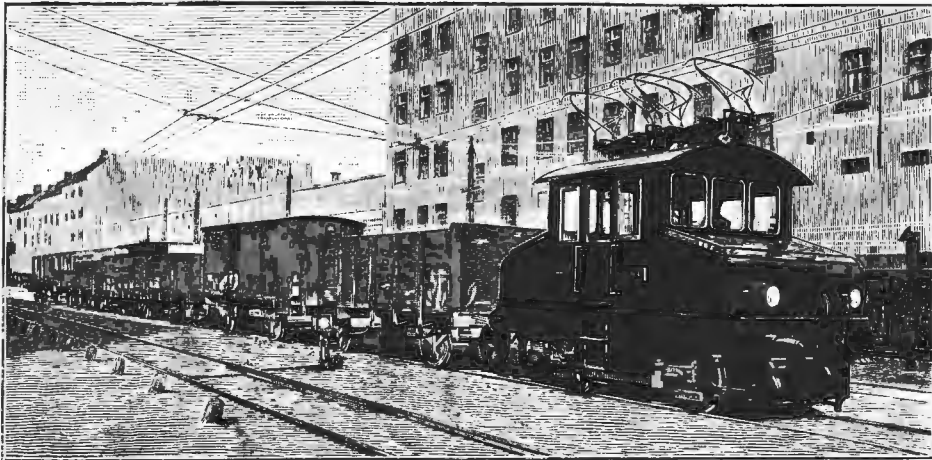
Новая электрическая желѣзная дорога для дальних сношеній. Рис. 1. Товарный поѣздъ. По фот. грав. Шайперъ.
