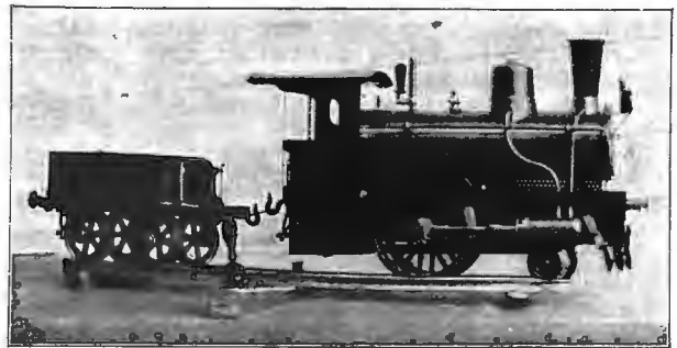
Рис. 51. Паровозъ новѣйшей конструкціи.
