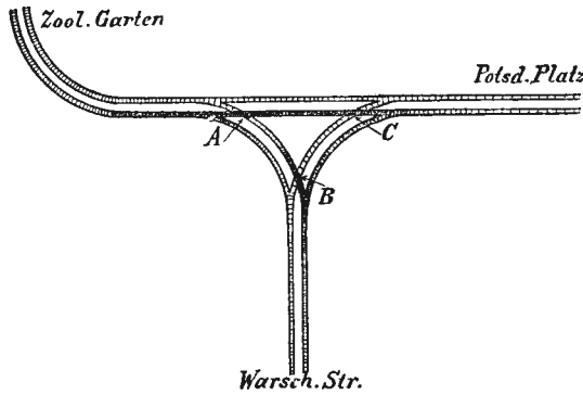
Рис. 2. Два параллельныхъ треугольника, образованныхъ расщепленіемъ рельсоваго пути.
