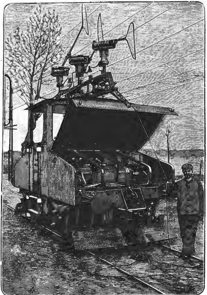
Новая электрическая желѣзная дорога для дальних сношеній. Рис. 2. Электрическая машина локомотива. По фот. грав. Шайперъ.
