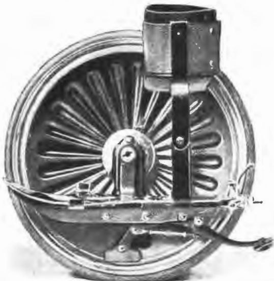
Коньки-колеса, изобретенные инж. Коллеромъ. Колесо, подставка для ноги, въ видѣ конька, и придѣланная къ ней на стержнѣ муфта, охватывающая икру ноги.
