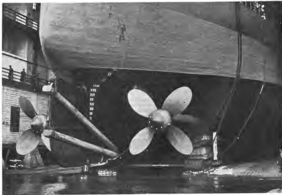
Спускъ броненосца „Императоръ Павелъ I“ 25 августа с. г. Броненосецъ въ докѣ Балтійскаго завода передъ спускомъ на воду. По фот. К. Булла авт. «Нивы».
