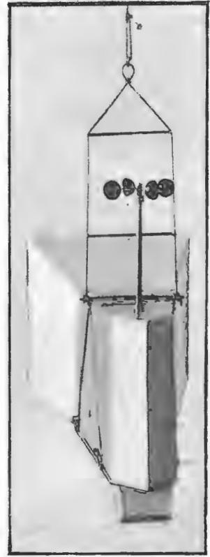
Метеорографъ системы В. В. Кузнецова, заключенный въ коробку и подвѣшенный къ змѣю.
