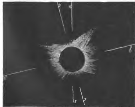
Видъ солнечной короны. (По Ганскому). а в—направленіе солнечнаго затмения.
