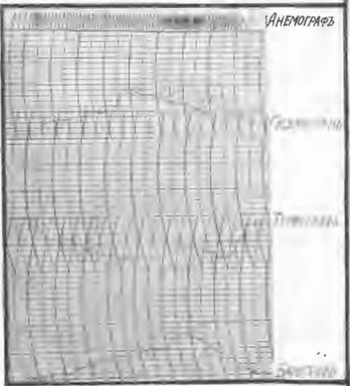
Запись метеорографа системы В. В. Кузнецова. Анемографъ — скорость вѣтра, гидрографъ — влажность, термографъ — температура, барографъ — давленіе воздуха.
