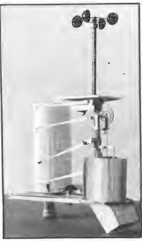
Общій видъ устройства метеорографа В. В. Кузнецова.
