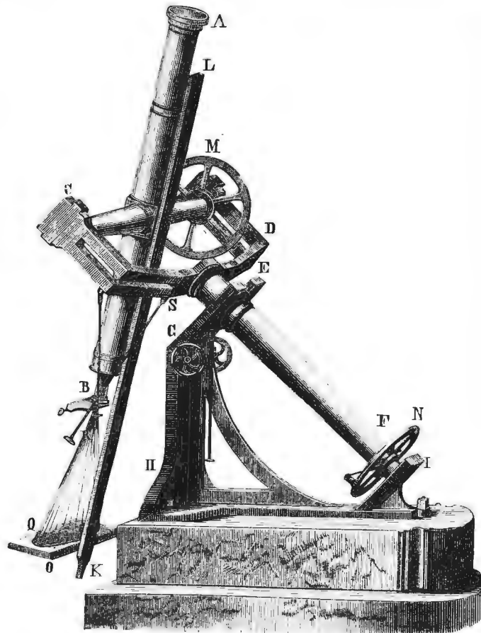
Фото-телескопъ Сенни. Грав. М. Рашевскій.
