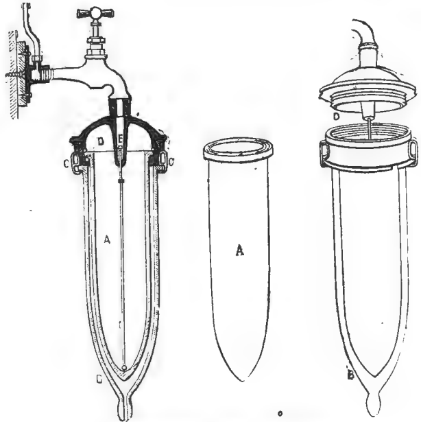
Аэро-фильтръ. Фиг. 2. Разрѣзъ.
