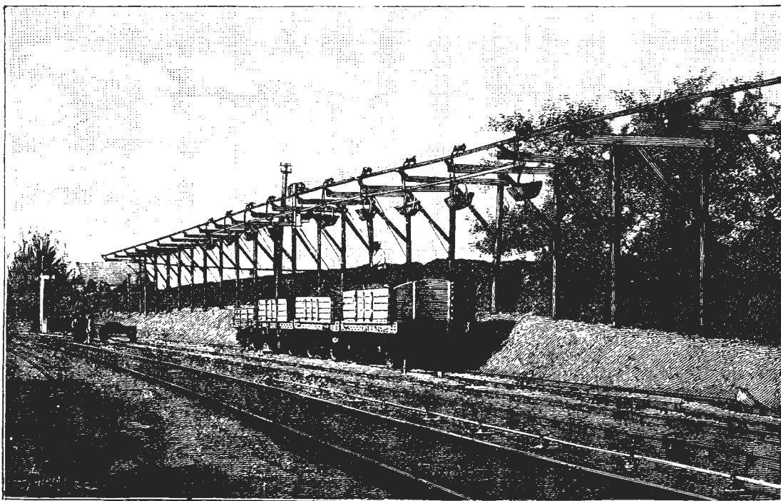
Фиг. 2. Мѣсто отправленія тельферной линии въ Глэндъ, въ Англии. По фотогр. грав. Тирія.
