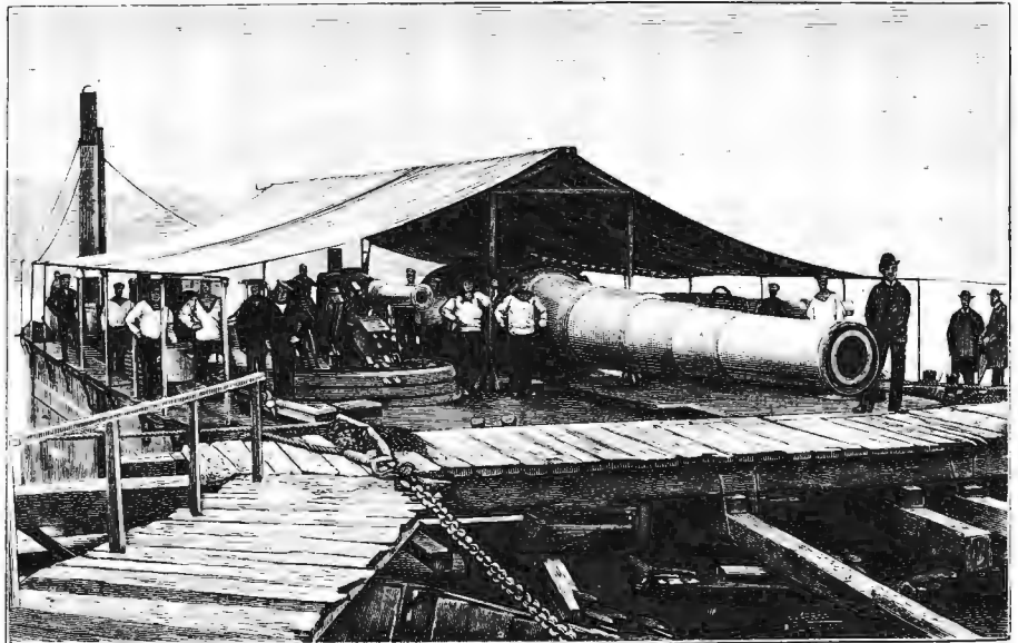
Шеститысячепудовое (100 тоннъ) орудіе на понтонѣ „Валента“.
