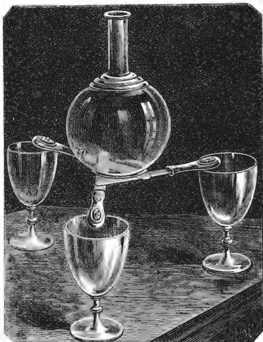
Физическіе опыты. Фиг. 2. Опытъ равновѣсія съ тремя ножами.
