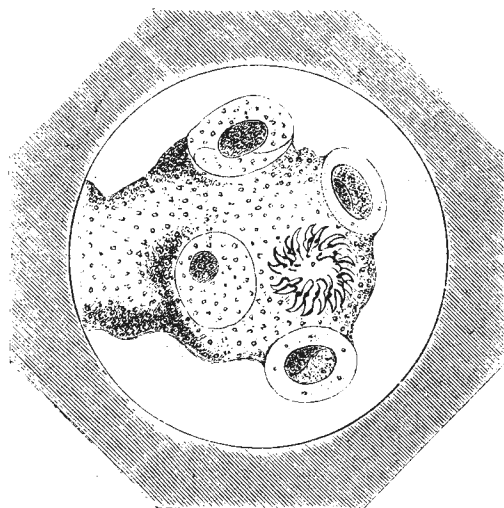
Подъ микроскопомъ. (Рис. 8). Крупки. (Стр. 462).
