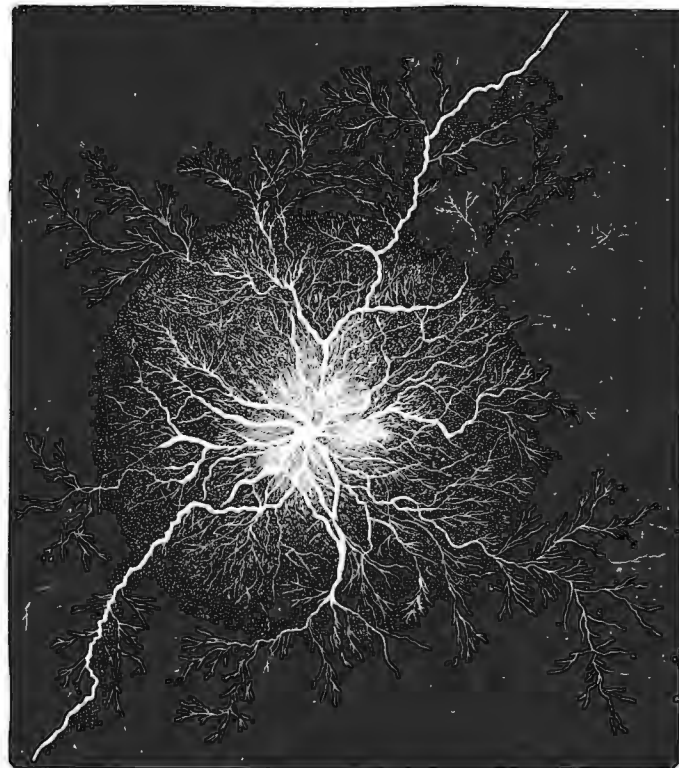
Моментальная фотографія электрической искры во время удара ея въ металлическую поверхность.
