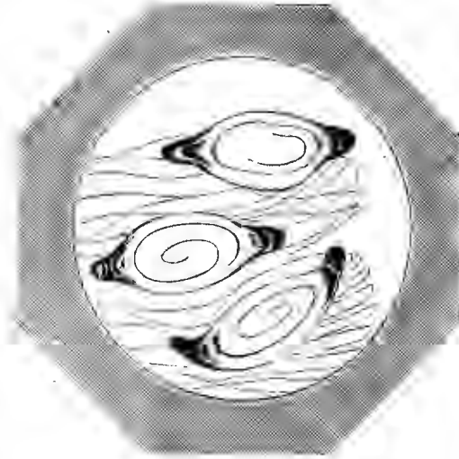
Подъ микроскопомъ. (Рис. 6). Капсулы трихинъ.
