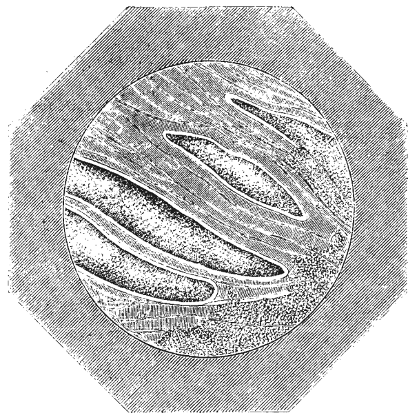
Подъ микроскопомъ. (Рис. 7). Мышечный псороспермій.
