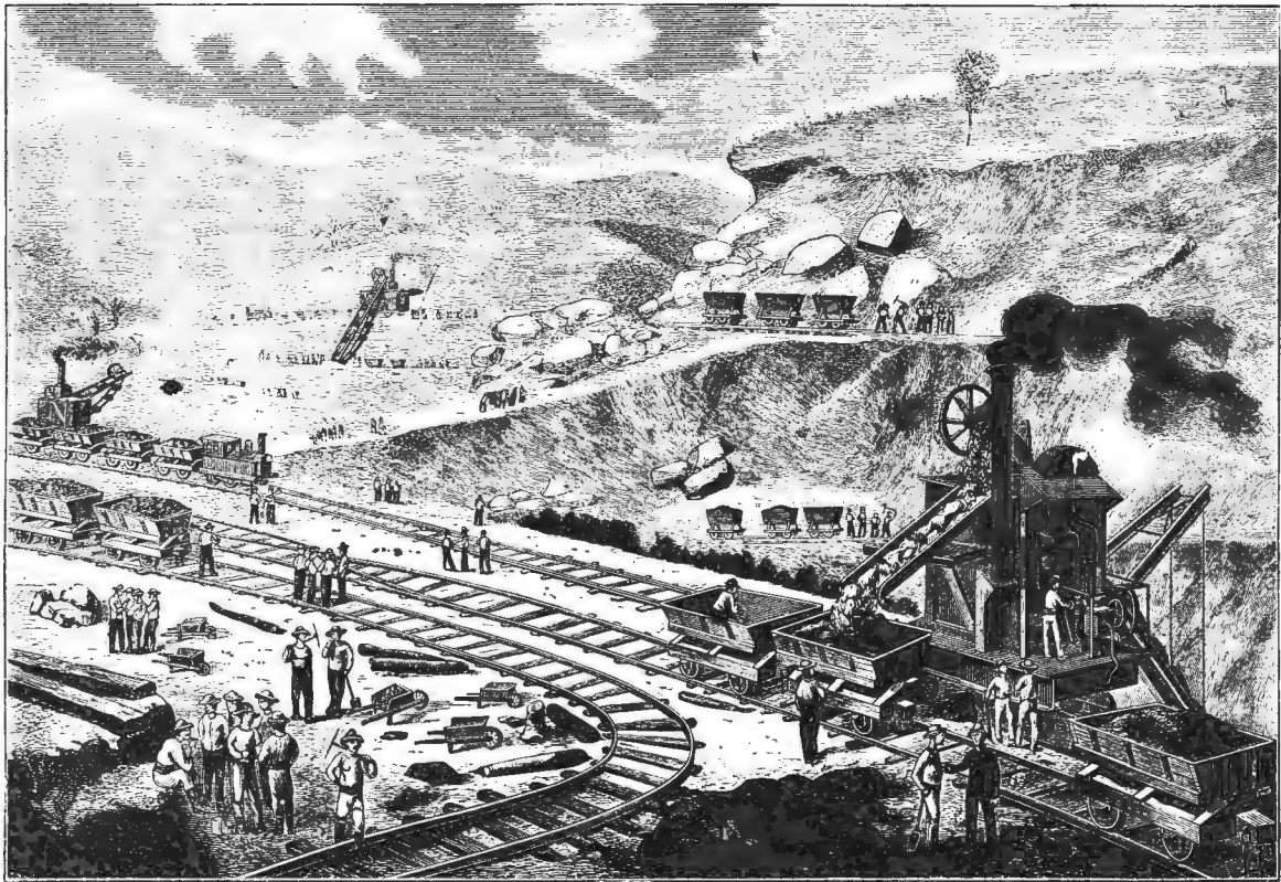
Работы на Панамскомъ каналѣ. Большія землекопныя машины (экскаваторы) на Императорскомъ участіи.
