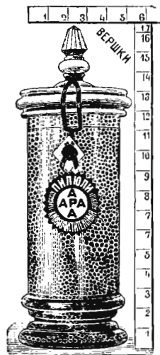
Размѣры банки внутри: Разрѣзъ въ серединѣ: диаметръ 4 3 / 8 верш. Высота 11 7 / 16 верш.
