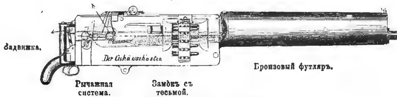
Фиг. 1. Главныя части митральезы Максима.
