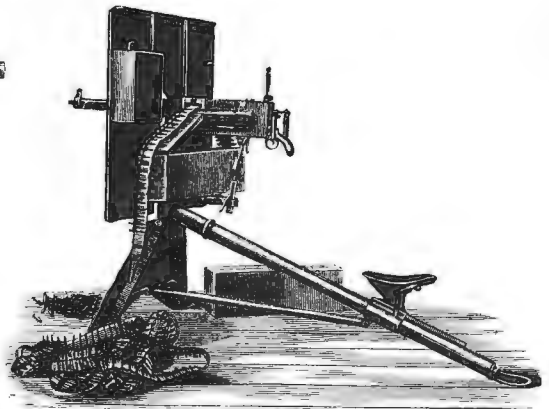
Фиг. 3. Митральеза съ треножникомъ и стальнымъ щитомъ.
