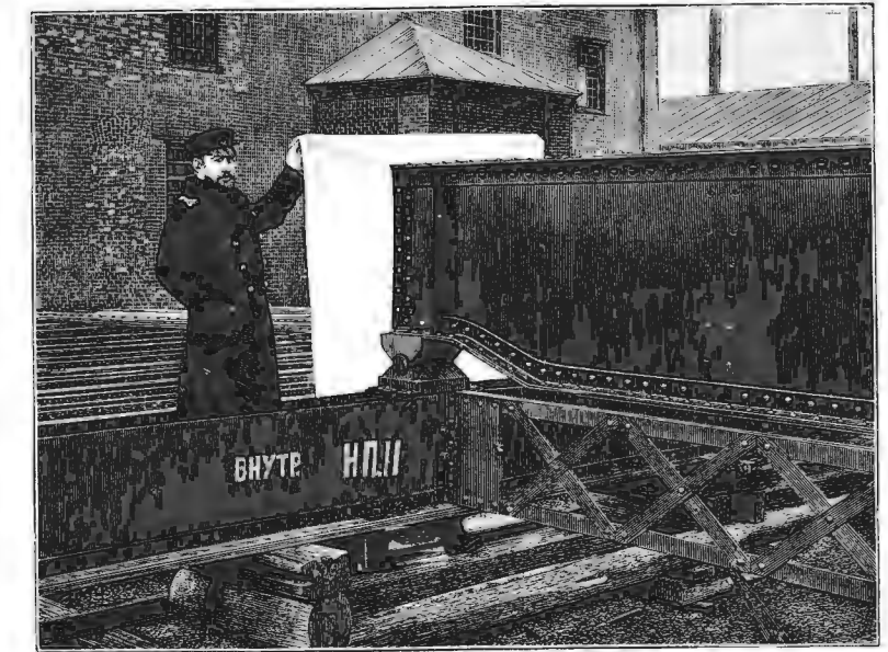
Деталь устройства свободной поперечной балки (мосты чрезъ Бѣлю, Уфу и Волгу у Твери). Съ фотогр. грав. М. Рашевскій.
