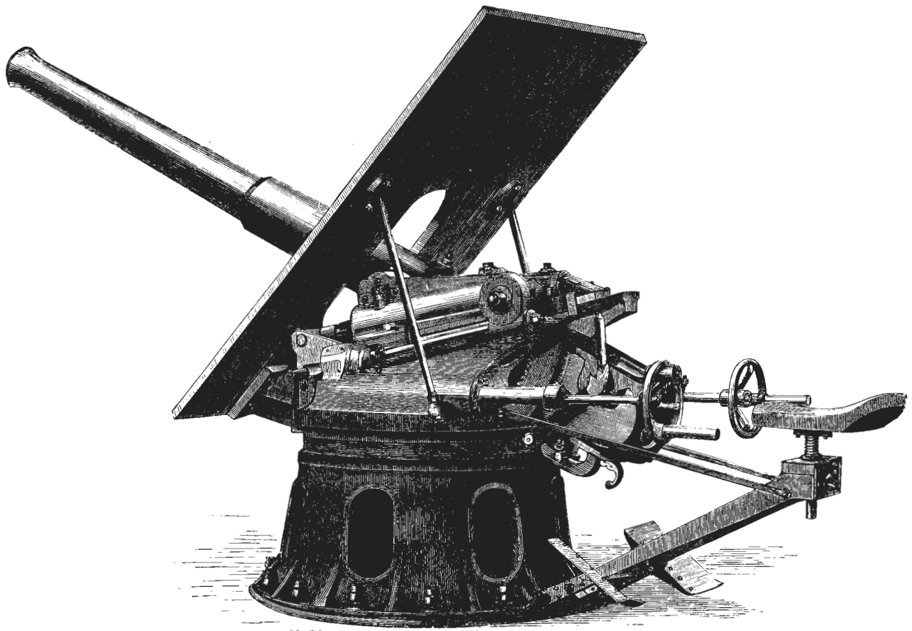
Новая скорострѣльная пушка Круппа.
