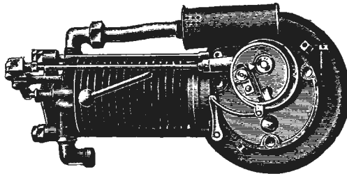
Велосипедъ-автомобиль. Моторъ Клемана.
