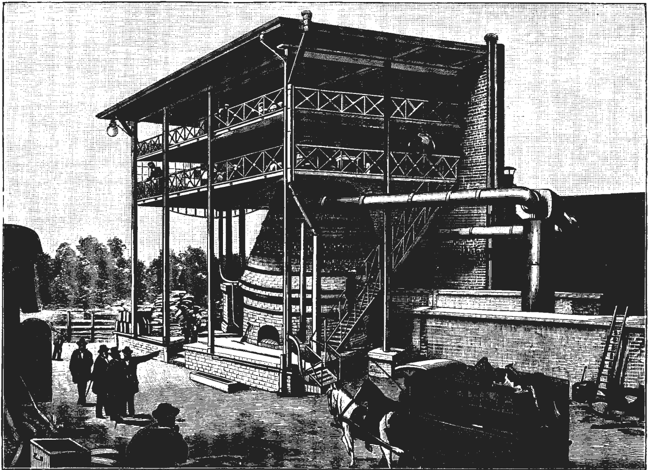
„Цѣнный мусоръ“. Печь для сжиганія мусора въ Берлинѣ. По фот. грав. Шюблеръ.
