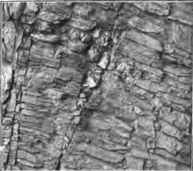
Гранитный слой съ гнѣздами аметистовъ въ трещинахъ.
