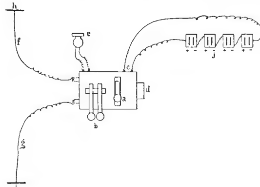
a) ключ; b) кнопки; c) зажимные винты; d) расщепитель; e) телефон; f, g) проволоки, ведущие к медным пластинкам в земле; h, i) медные пластинки в земле; j) батареи.
