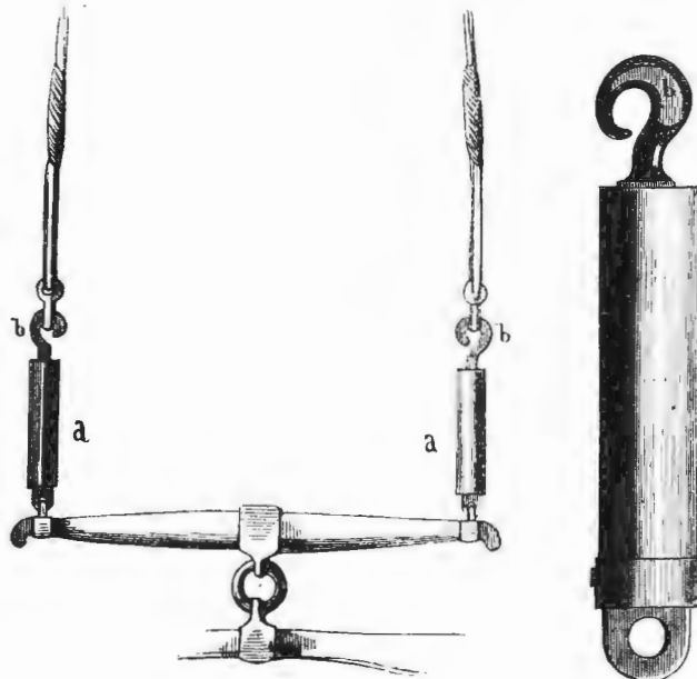
Фиг. 1. Фермановъ аппаратъ для сбереженія лошадиной силы. Грав. Вейерманъ. Фиг. 2.
