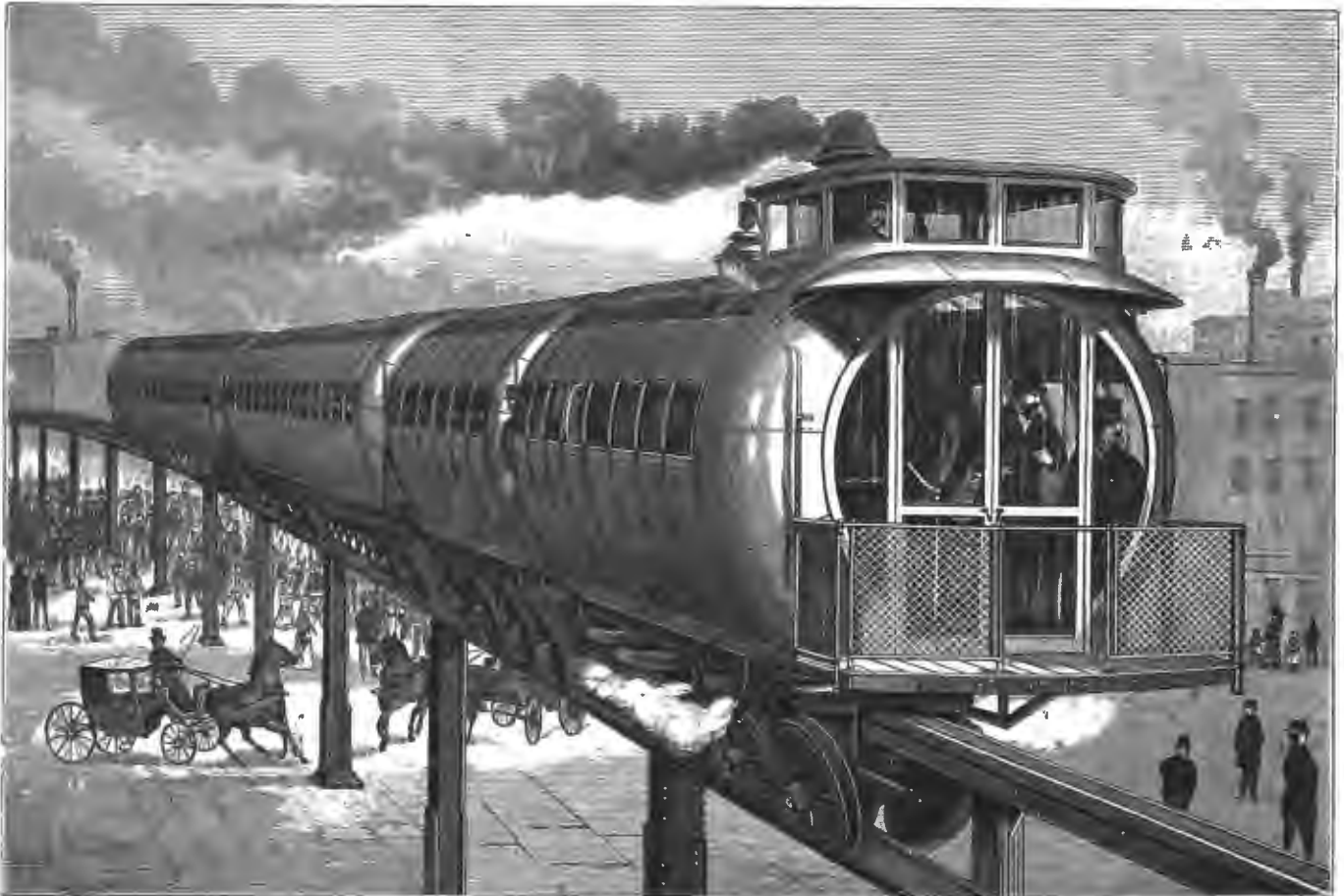
Городская желѣзная дорога на столбахъ въ Бостонѣ. По рис. съ натуры, грав. Дж.
