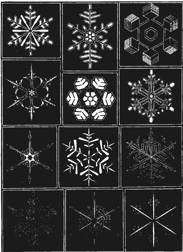
Рис. 1. Снѣжные кристаллы, по изображенію Глешера (1859 г.).
