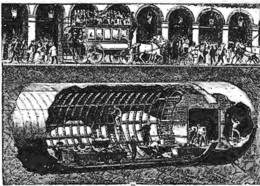
Проектъ подземной жел. дор. въ Парижѣ. Проложеніе пути.
