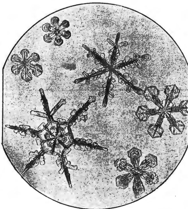
Рис. 6. Снѣжные кристаллы по увеличеннымъ въ 20 разъ фотографическимъ снимкамъ д-ра Нейгауза
