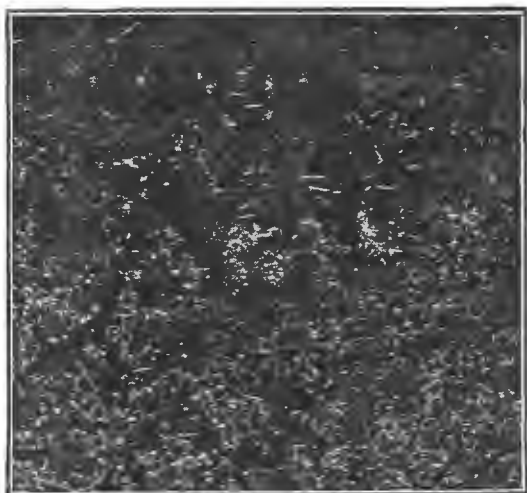
Рис. 13. Кругообразные кристаллоиды, полученные на стеклѣ, поцарапанномъ пескомъ.
