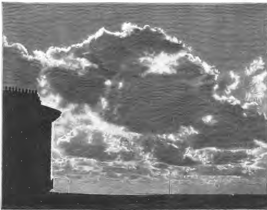
Рис. 3. Cumulus — кучевая облака.
