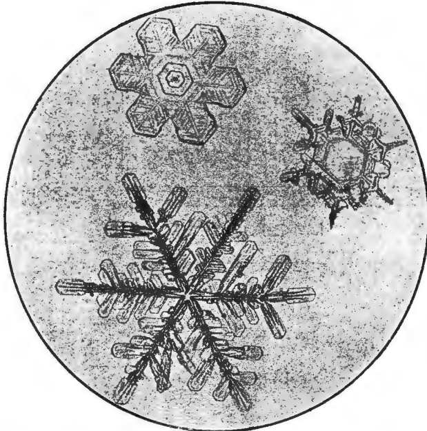
Рис. 8. Снежные кристаллы по увеличенным в 20 раз фотографическим снимкам д-ра Нейгауза.
