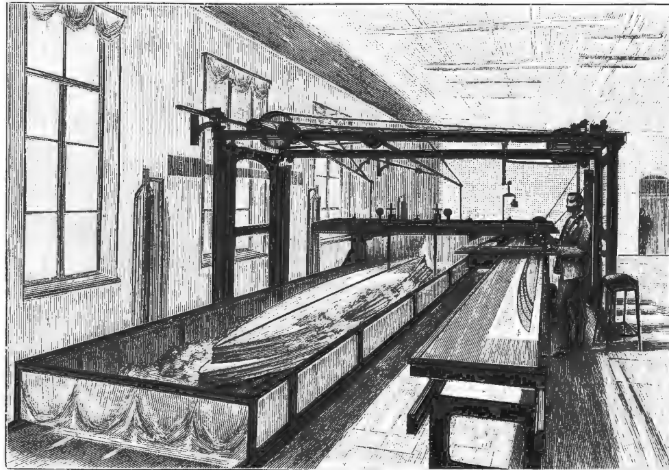
Моделе-стругательный станокъ при бассейнѣ для опредѣленія сопротивленія воды при движеніи моделей судовъ. Рис. Г. Бролинга, грав. Рашевскій.
