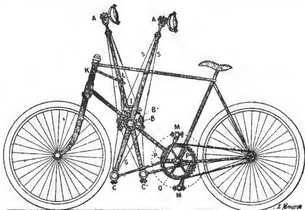
Система бициклета.
