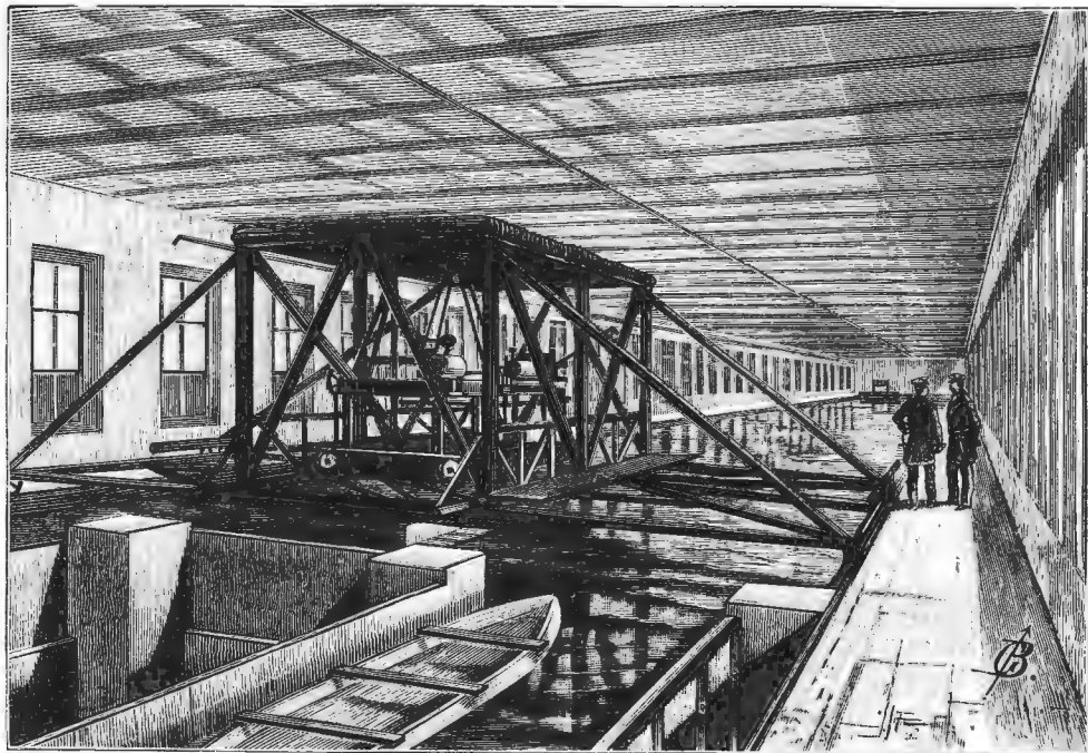
Бассейнъ для опредѣленія сопротивленія воды при движеніи моделей судовъ и динамометрическая тѣлѣжка. Рис. Г. Бролинга, грав. Рашевскій.
