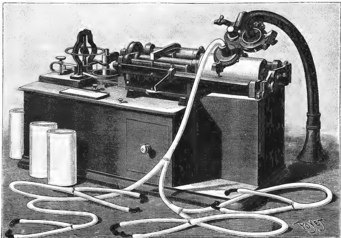
Новый фонографъ Эдисона.
