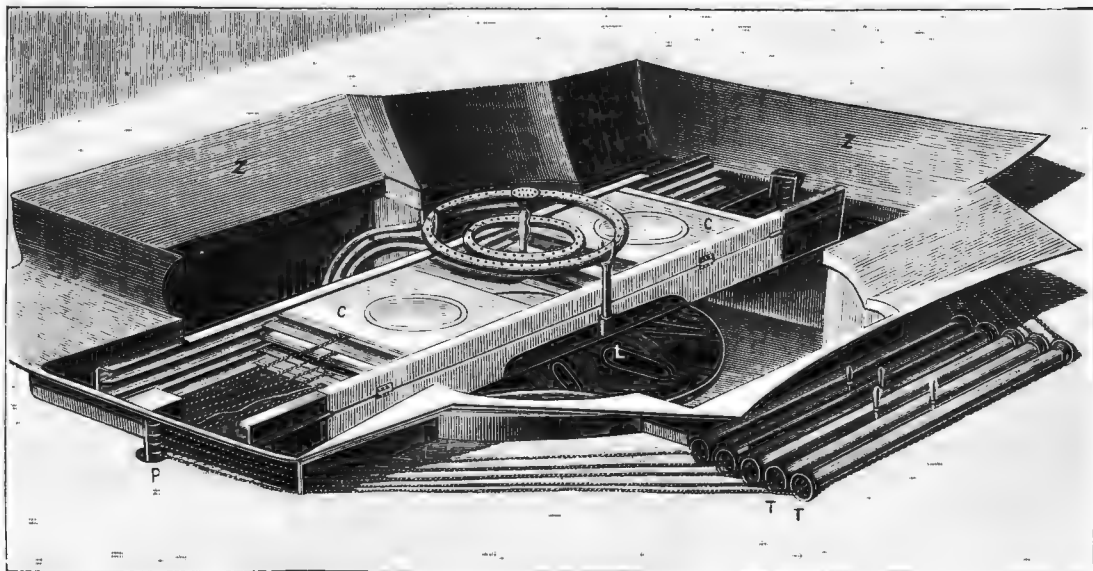
Механизмъ свѣтящагося фонтана Гастона Менъе.
