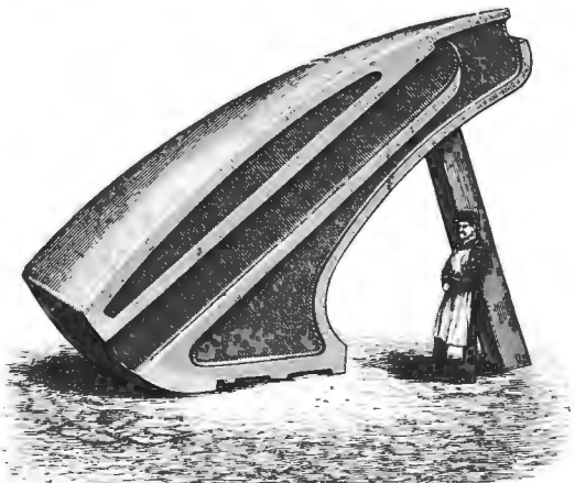
Рис. 2. Панцирная броня для опытовъ стрѣльбы въ Спощи (1886).
