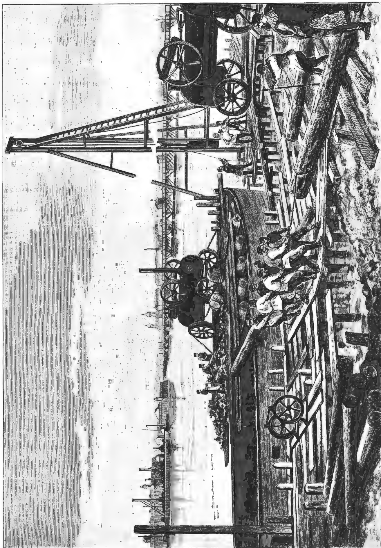
Предварительная работа для перемещения Троицкого моста в СПб. на новое место, против Мраморного переулка. Ориг. рис. Броллинга, грав. Рапеевский.
