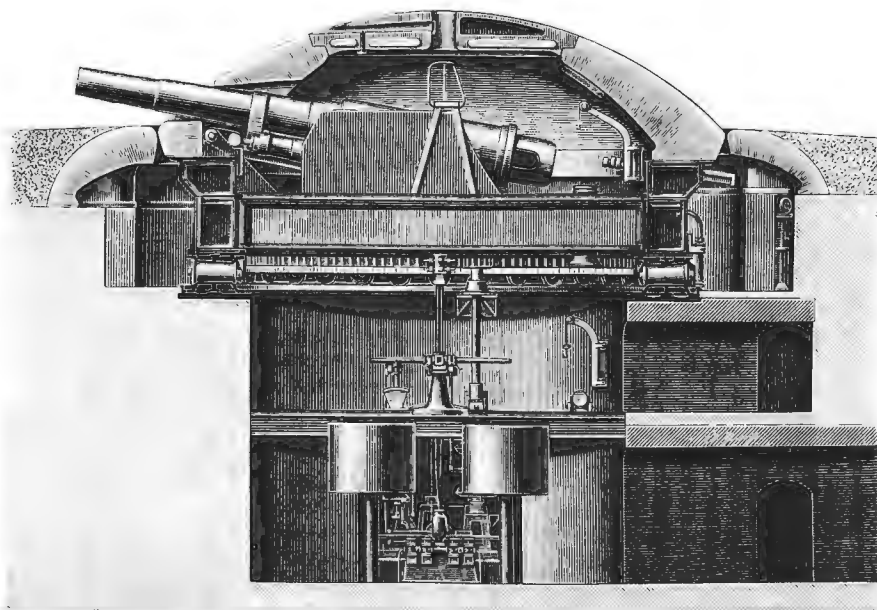
Рис. 4. Внутренній видъ панцирной башни для двухъ 30,5-центиметр. пушекъ съ машинами и ручнымъ приводомъ.
